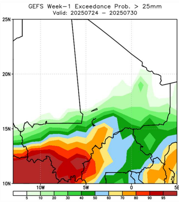
Probabilité S_1 > 25\text{mm}
