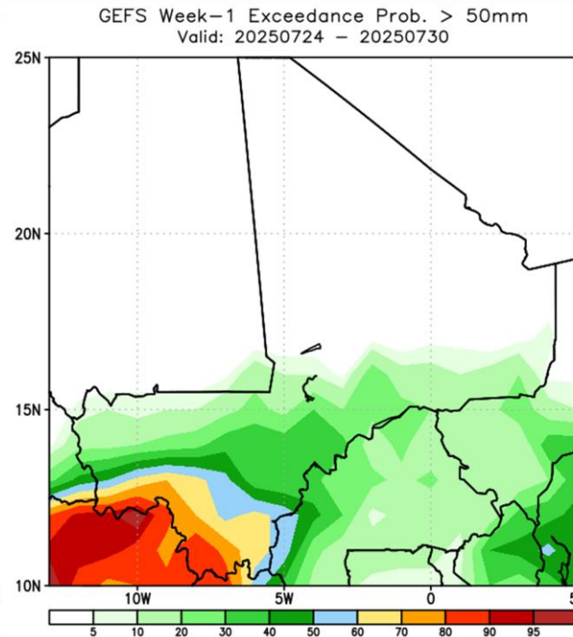
Probabilité S_1 > 50\text{mm}
