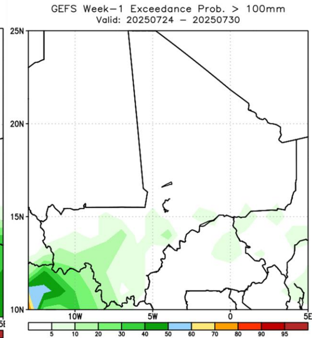
Probabilité S_1 > 100\text{mm}
